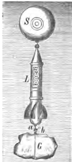
Č. 476. Bathometr Roussetův.
